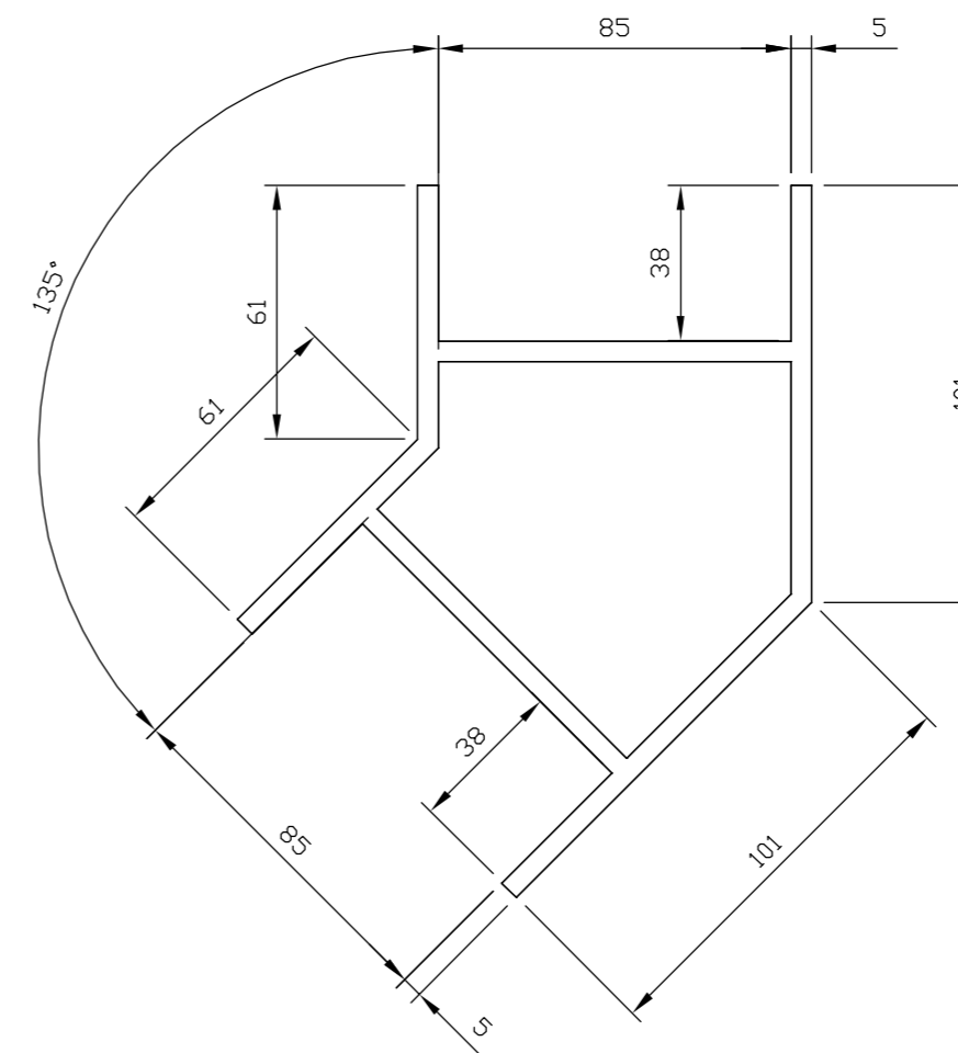
STD 45° CORNER L-121019-RAW-DT-05
